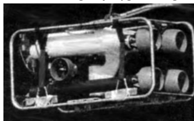
Undervattensfarkosten Sjugglan
